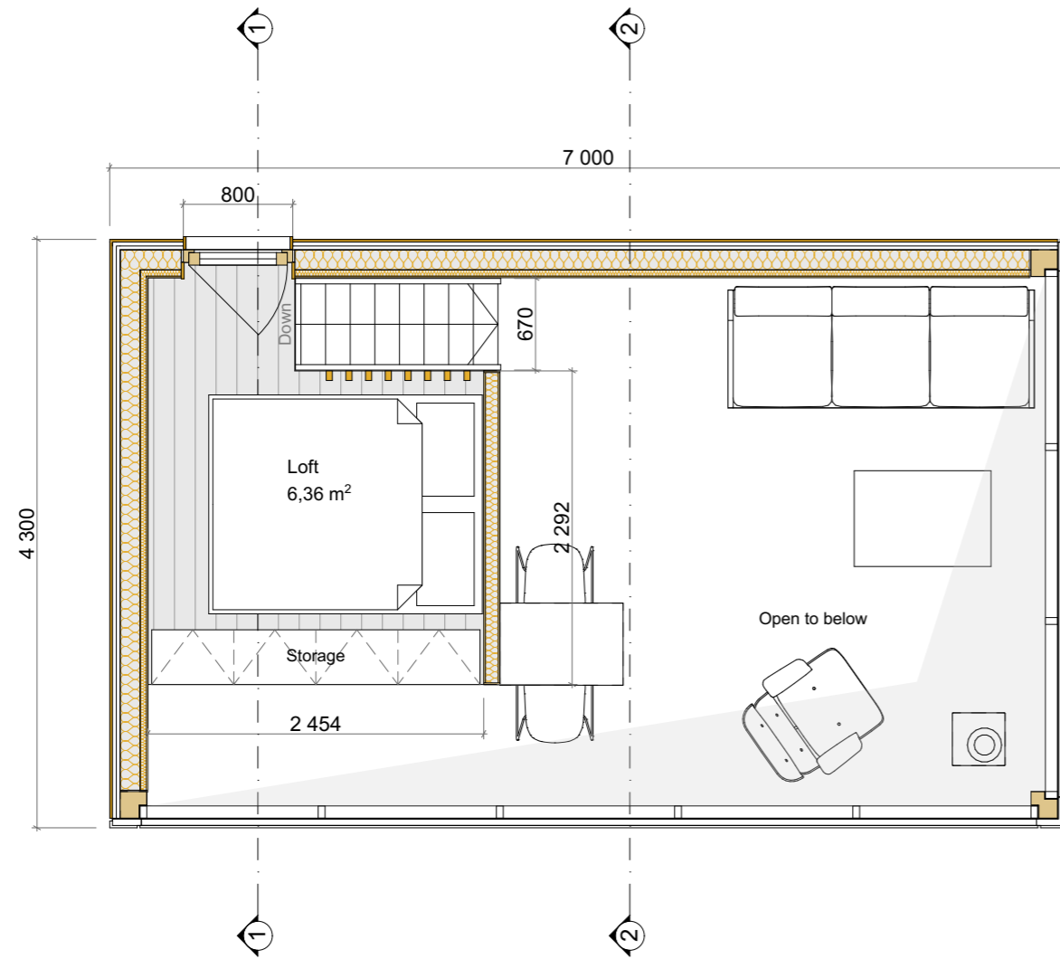
PLAN 2,24 M 1:50
